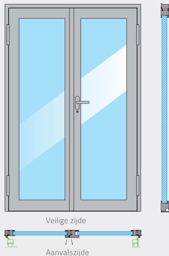
DUBBELE DRAAIDEUR - BEGLAASDE VERSIE
