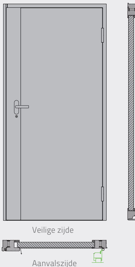
ENKELE DRAAIDEUR - VOLLE VERSIE MET VLAK PLAATWERK
