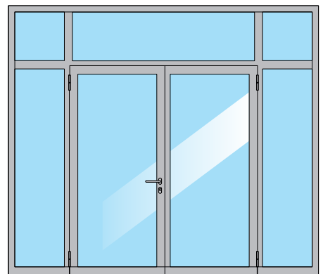
INBOUW VAN EI1-30 DUBBELE DEUR IN VASTE SCHEIDINGSWAND MET EI30-BEGLAZING
